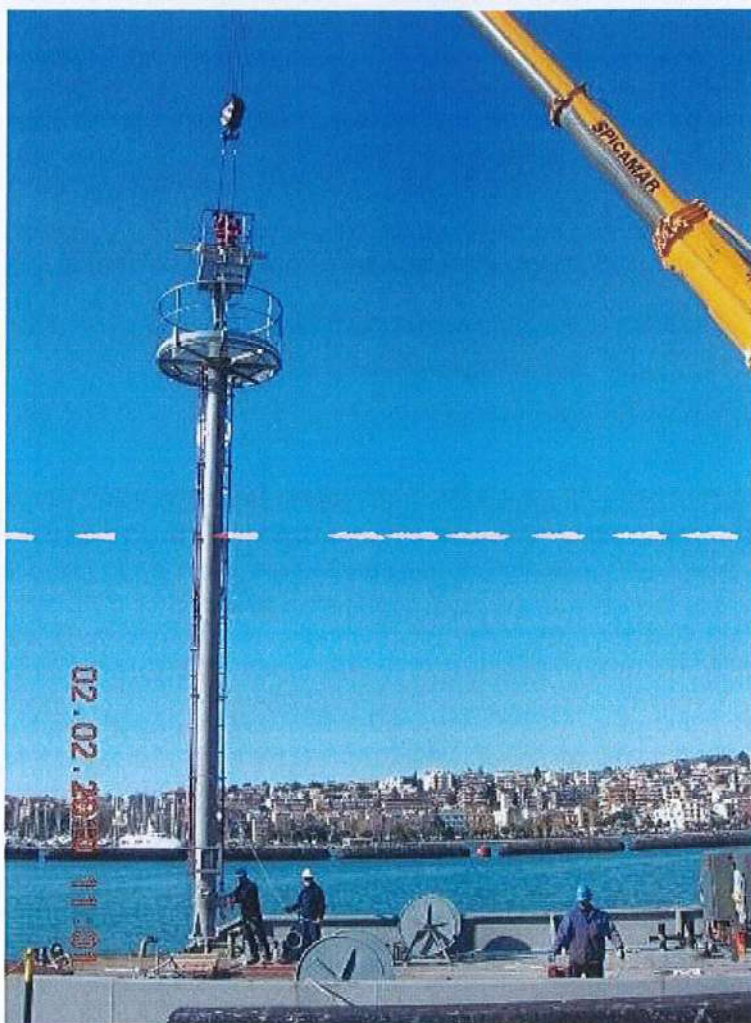
GAETA (LT) - FASE DI MONTAGGIO DI UNA DELLE DUE TORRI ANTINCENDIO
